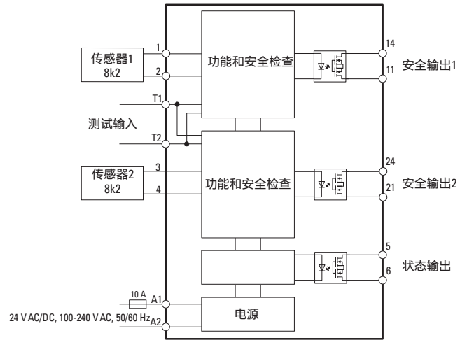
电路图
